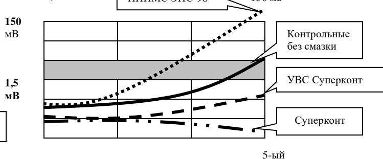
Рис2. Изменение падения напряжения на контактах медь-алюминий при увеличении температуры до 300 °С после 5 циклов нагревание-охлаждение. Плотность рабочего тока 0,4 А/мм 2
