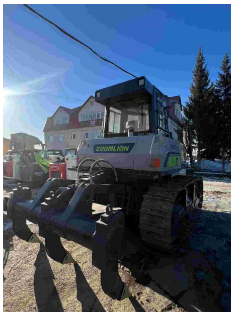
Гусеничный Бульдозер Zoomlion ZD 170-3 с трехзубым рыхлителем
